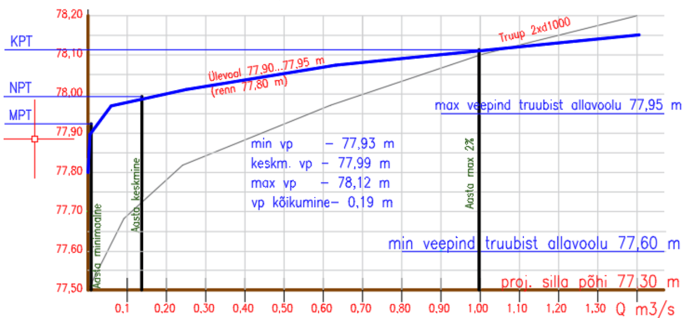
Joonis 6 Variant 2 - Ülevoolu graafik
