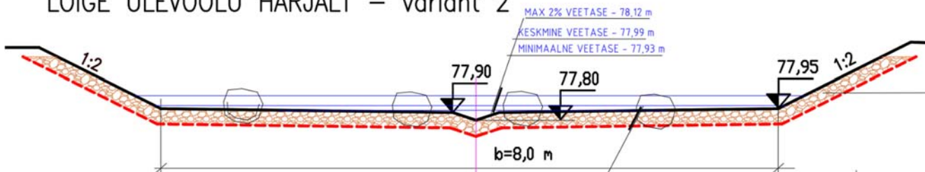
Joonis 5 Variant 2 - Lõige kärestiku ülevoolu harjalt
