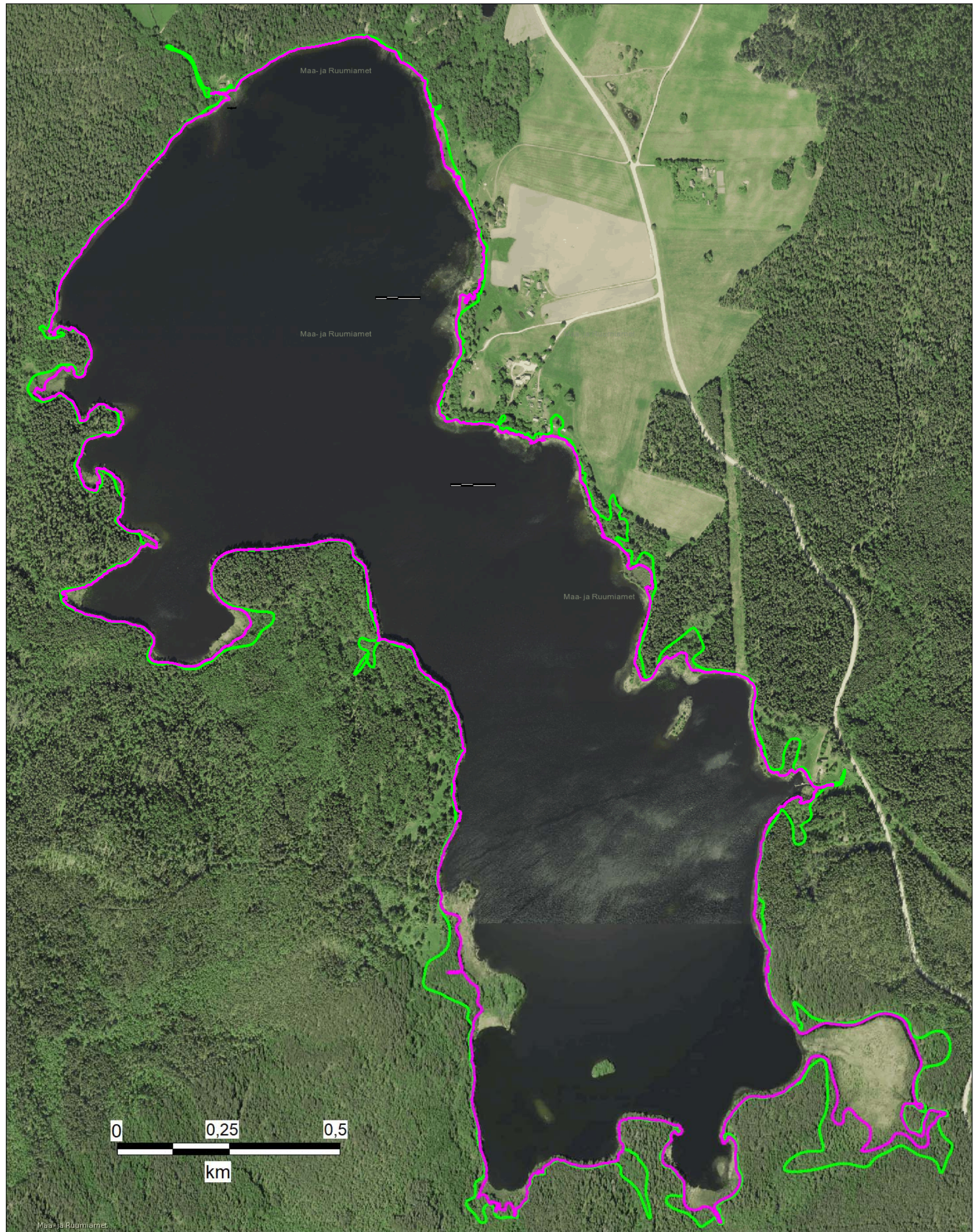
Joonis 9 Maapinna kõrgusjooned järve ümber (lilla 78,00 m, roheline 78,20 m)
